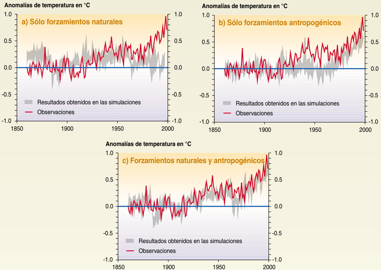
Figura RRP-2: La simulación de la variación de temperaturas (°C) y la comparación de los resultados con los cambios registrados nos permiten comprender mejor las causas que producen los principales cambios.
