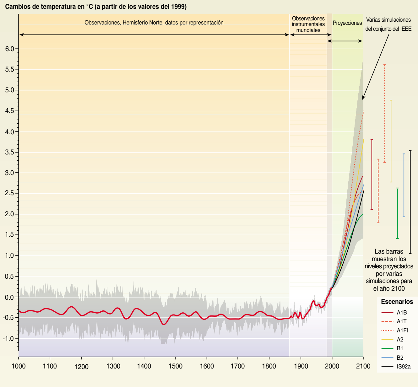
Figura RRP-10b: Se muestran las variaciones en la temperatura media de la superficie en el Hemisferio Norte durante el periodo 1000–1860 (no se dispone de los datos correspondientes para el Hemisferio Sur) extraídos a partir de datos por representación (anillos de los árboles, corales, testigos de hielo y registros históricos). La línea muestra una media en 50 años, el área gris, el límite de confianza del 95 por ciento en los datos anuales. Para el periodo 1860–2000 se muestran las observaciones de variaciones anuales y mundiales de la temperatura media de la superficie obtenidas del registro instrumental. La línea muestra la media por decenios. Para el periodo 2000–2100, se muestran las proyecciones de la temperatura media mundial de la superficie para los seis escenarios ilustrativos del IEEE y los del IS92a, estimadas mediante una simulación con sensibilidad climática media. El área gris marcada 'Varias simulaciones del conjunto del IEEE' muestra la gama de resultados de los 35 escenarios del IEEE además de aquellos obtenidos de una gama de simulaciones con diferentes sensibilidades climáticas. La escala de temperaturas se determina a partir del valor para 1990; la escala es diferente de la utilizada en la Figura RRP-2.
