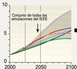
(j) Forzamiento radiativo ( Wm^{-2} )
