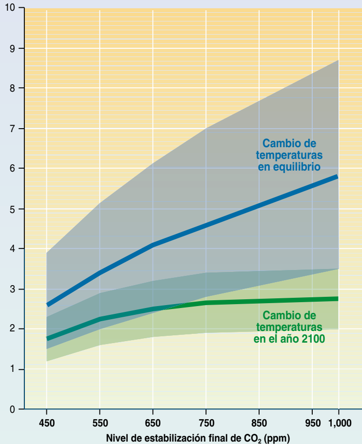
Figura RRP-7: Las concentraciones de CO 2 para la estabilización podrían disminuir el calentamiento, pero en un grado incierto. Los cambios de temperatura con relación a 1990, mostrados en a) el año 2100, y b) en equilibrio, se estiman sobre la base de una simulación climática sencilla para los perfiles WRE, como en la Figura RRP-6. Las estimaciones mínimas y máximas para cada nivel de estabilización suponen una sensibilidad climática de 1,7 y 4,2°C respectivamente. La línea central es una media de las estimaciones máximas y mínimas.
