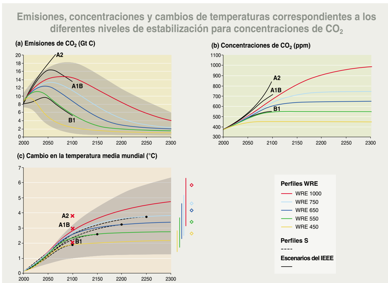
Figura RRP-6: La estabilización de las concentraciones de CO 2 requeriría una reducción importante de las emisiones por debajo de los niveles actuales, y frenaría la velocidad del calentamiento.
