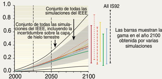
(I) Elevación del nivel del mar (m)
