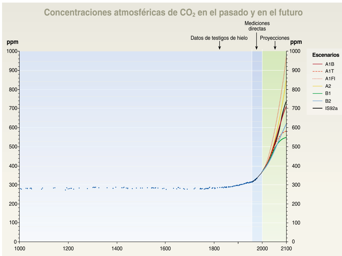
Figura RRP-10a: Concentraciones atmosféricas de CO 2 desde el año 1000 al 2000 a partir de datos de testigos de hielo y mediciones atmosféricas directas durante los últimos decenios. Las proyecciones sobre concentraciones de CO 2 durante el período 2000–2100 están basadas en los seis escenarios del IEEE y el IS92a (para compararlos con el SIE). P9 Figura 9-1a
