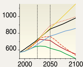
(d) Emisiones de N 2 O (Tg N)
