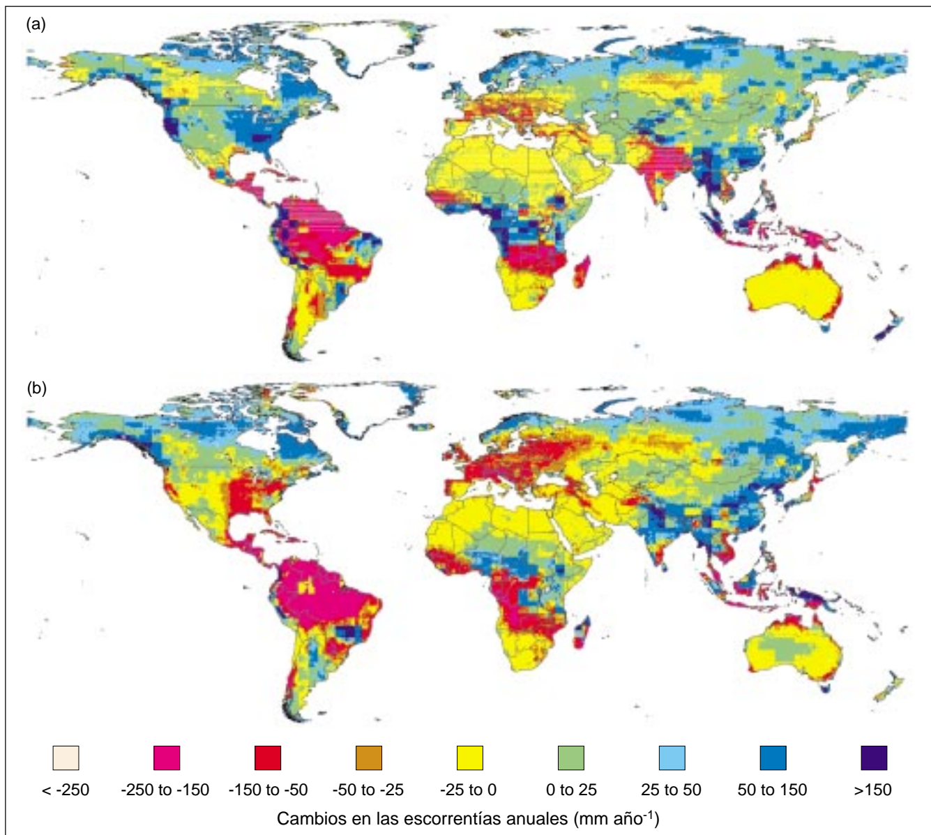
Figura SMP-4: Los cambios proyectados en la cantidad media anual de escorrentía para el año 2050, en relación con la cantidad media de escorrentías de los años 1961–1990, siguen en gran medida los cambios proyectados en las precipitaciones.
